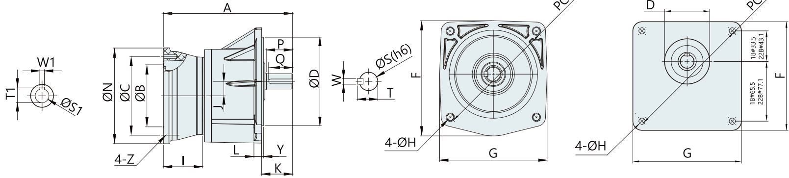
A型法蘭 (框號 22、28、32用)
