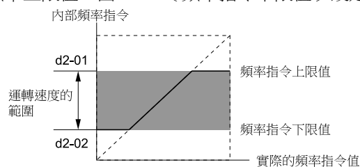
圖 11.58 頻率指令上限/下限
