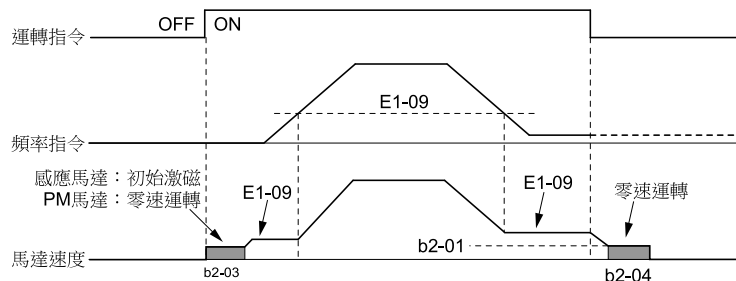
圖 11.20 最低輸出頻率下的運轉
