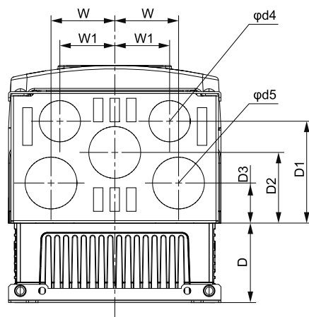
圖 9.6 外形圖2 (型號：2056、4031、4038)
