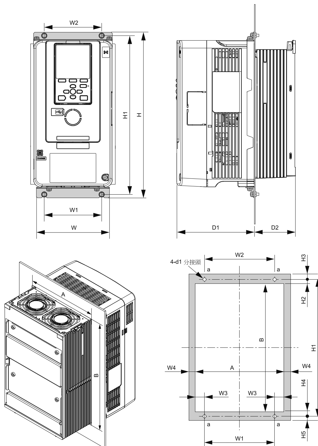
圖 2.27 開孔尺寸
