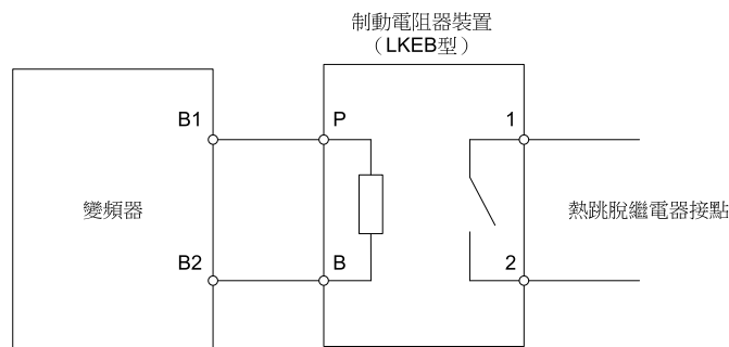
圖 2.61 制動電阻器裝置（LKEB型）的連接（例如：2004~2138、4002~4168）
