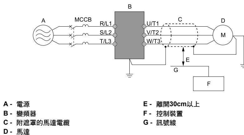
圖 2.70 感應干擾防止對策
