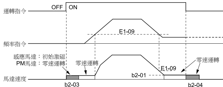
圖 11.21 零速運轉
