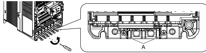
A - 保護蓋安裝螺絲
