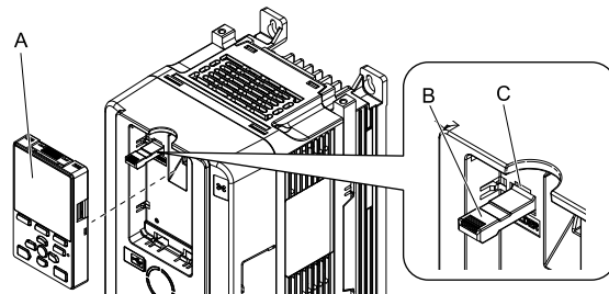
A - 操作器 B - 操作器介面 C - 插座
