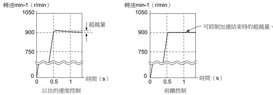
圖 11.139 透過前饋控制的超越量的抑制
