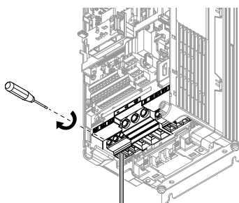
圖 2.40 緊鎖端子台的螺絲
