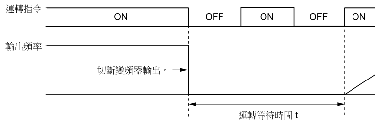
圖 11.16 附定時的自由運轉停止
