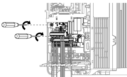
圖 7.28 固定端子台
