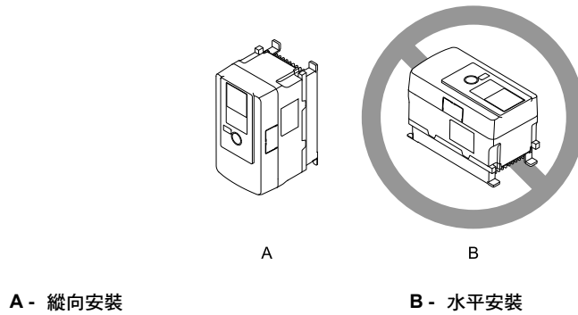
圖 2.1 安裝方向
