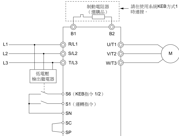
圖 11.126 KEB功能的配線範例
