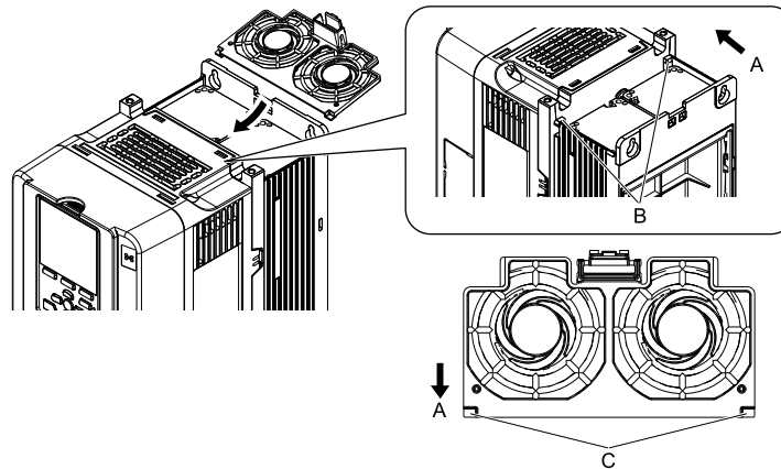
A - 變頻器正面 B - 鉤爪嵌入部
