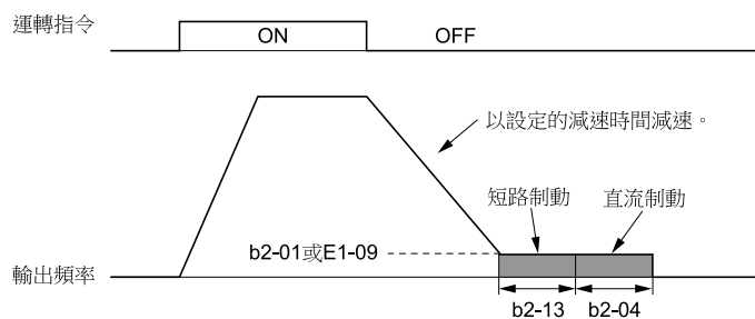
圖 11.11 PM用無PG向量控制、PM用無PG高級向量控制、EZ向量控制模式時的減速停止
