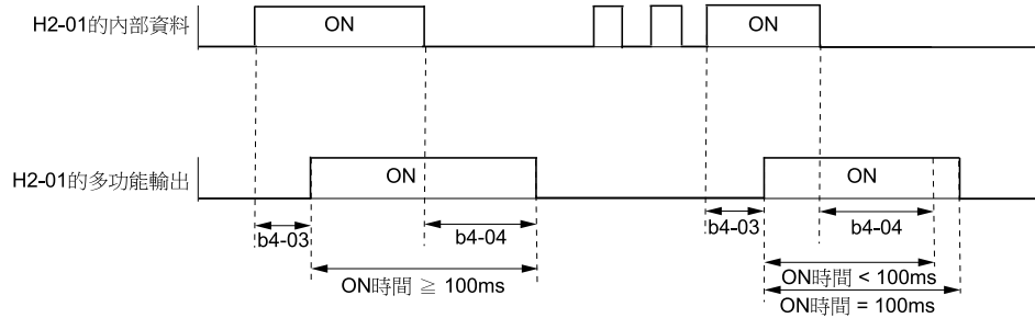
圖 11.33 使用H2-01端子的定時功能的動作範例
