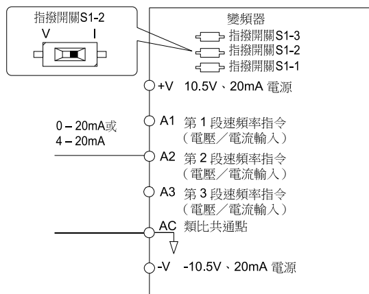
圖 11.9 在端子A2作為電流訊號設定頻率指令的範例
