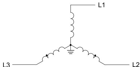
圖 4.7 對稱接地
