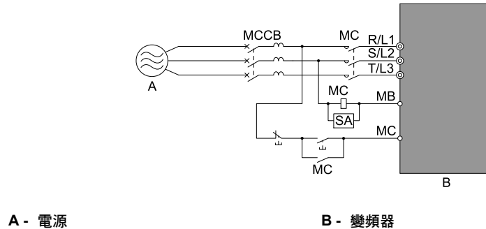
圖 2.65 配線用斷路器的連接
