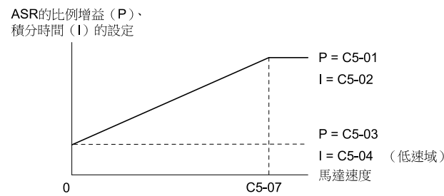
圖 11.53 低速/高速的增益設定
