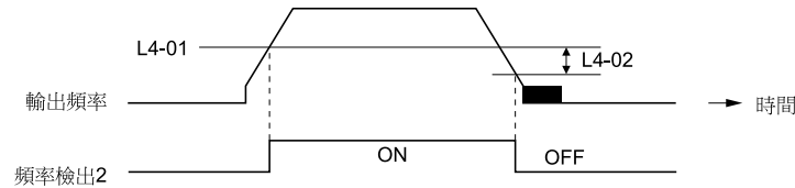
圖 11.1 頻率檢出2
