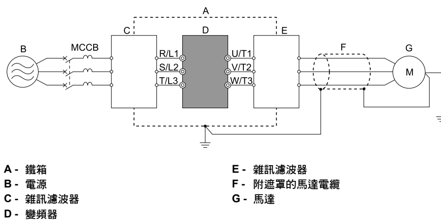
圖 2.71 無線電干擾防止對策
