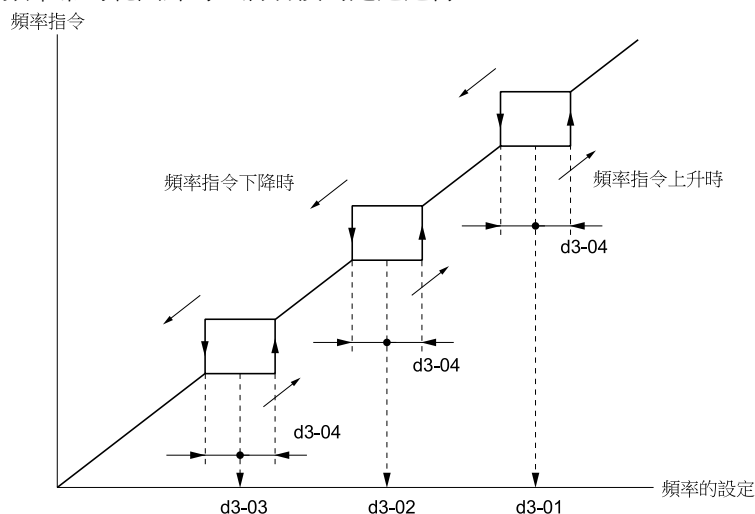
圖 11.59 跳躍頻率
