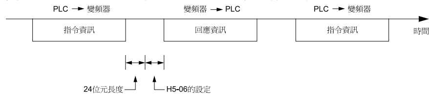
圖 5.5 回應等待時間
