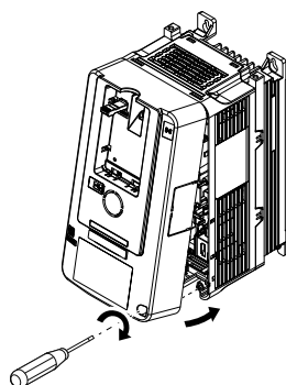
圖 2.21 安裝前外蓋
