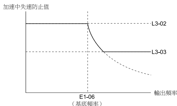
圖 11.130 加速中失速防止值/限制
