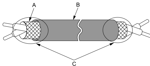
A - 將遮罩線連接在變頻器的端子E (G) 上。 B - 保護層 C - 用膠帶等進行絕緣。
