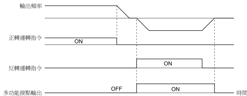
圖 11.95 反轉中輸出時序圖
