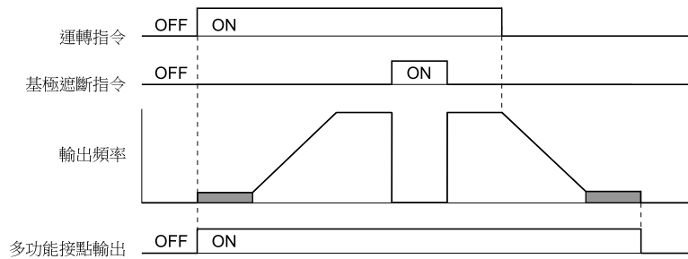
圖 11.85 運轉中的時序圖
