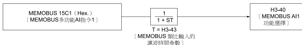
圖 11.101 MEMOBUS多功能AI指令1的功能區塊圖
