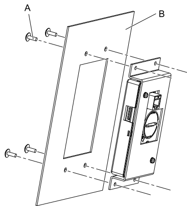
A - M4螺絲 B - 控制盤
