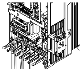
圖 2.51 控制迴路的配線
