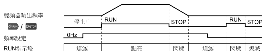
圖 3.7 RUN指示燈和變頻器動作的關係
