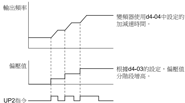
圖 11.64 UP2/DOWN2的偏壓值 (d4-03 ≠ 0.00Hz)
