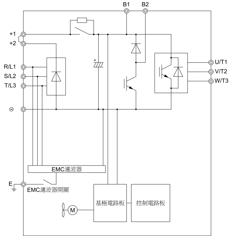
圖 2.33 變頻器的主迴路構成 ( 2004~2082 、 4002~4044 )
