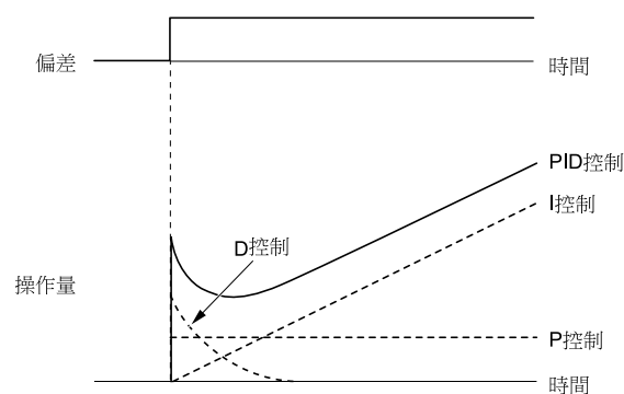
圖 11.34 PID控制的動作
