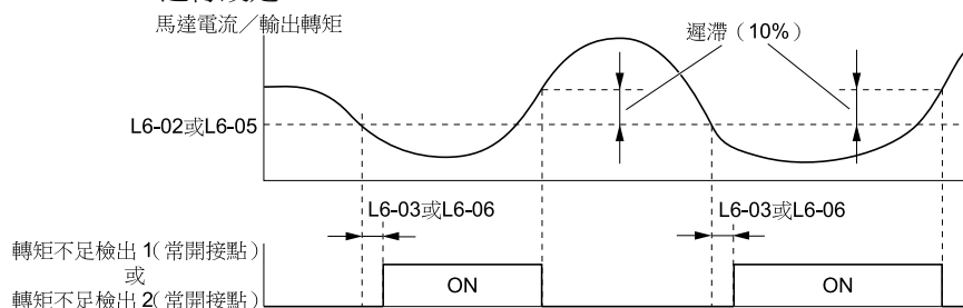
圖 11.135 轉矩不足檢出的時序圖
