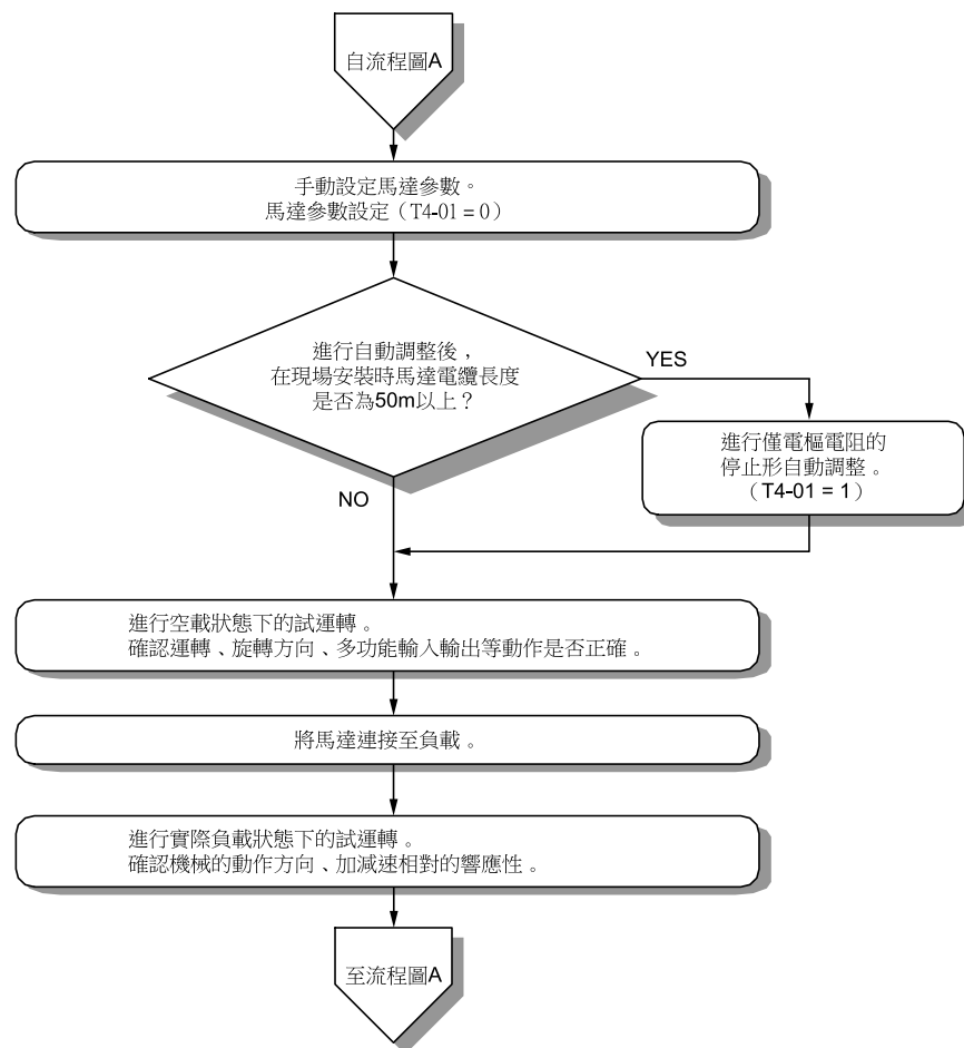
圖 3.11 EZ向量控制模式的試運轉步驟
