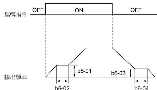
圖 11.40 起動時/停止時DWEELL功能的時序圖
