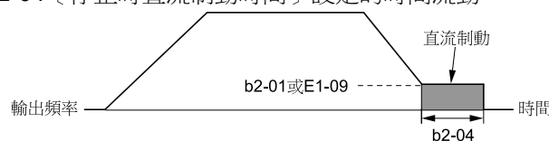
圖 11.24 停止時直流制動
