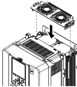
圖 7.16 安裝風扇外蓋
