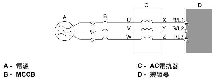
圖 2.66 AC電抗器的連接範例
