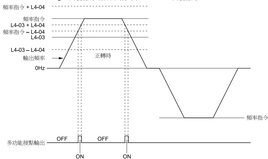
圖 11.92 任意頻率（速度）一致2的範例（L4-03為正時）
