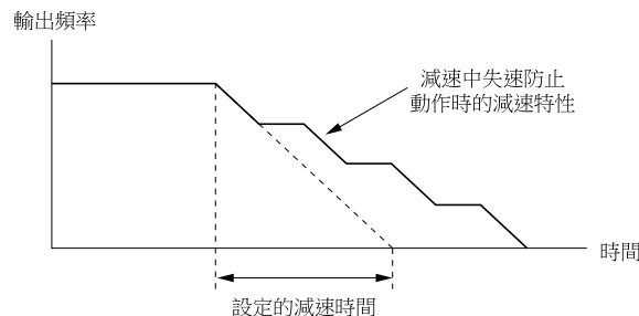
圖 11.131 減速中失速防止的動作範例
