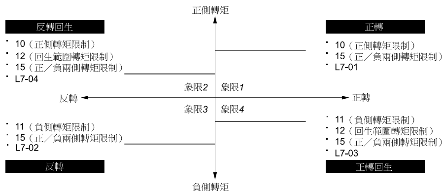
圖 11.106 轉矩限制和類比輸入的設定參數
