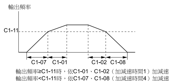
圖 11.46 加減速時間的切換頻率
