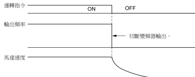
圖 11.13 自由運轉停止
