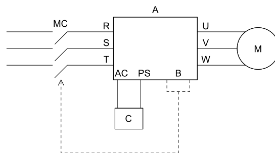
A - 變頻器 B - 多功能接點輸出端子
