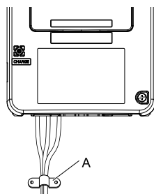
圖 7.20 安裝緊固扣
