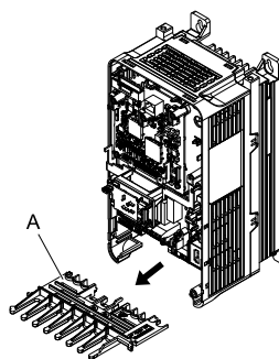
圖 2.38 拆下配線蓋
