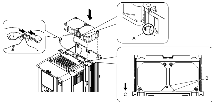
A - 風扇的開口
