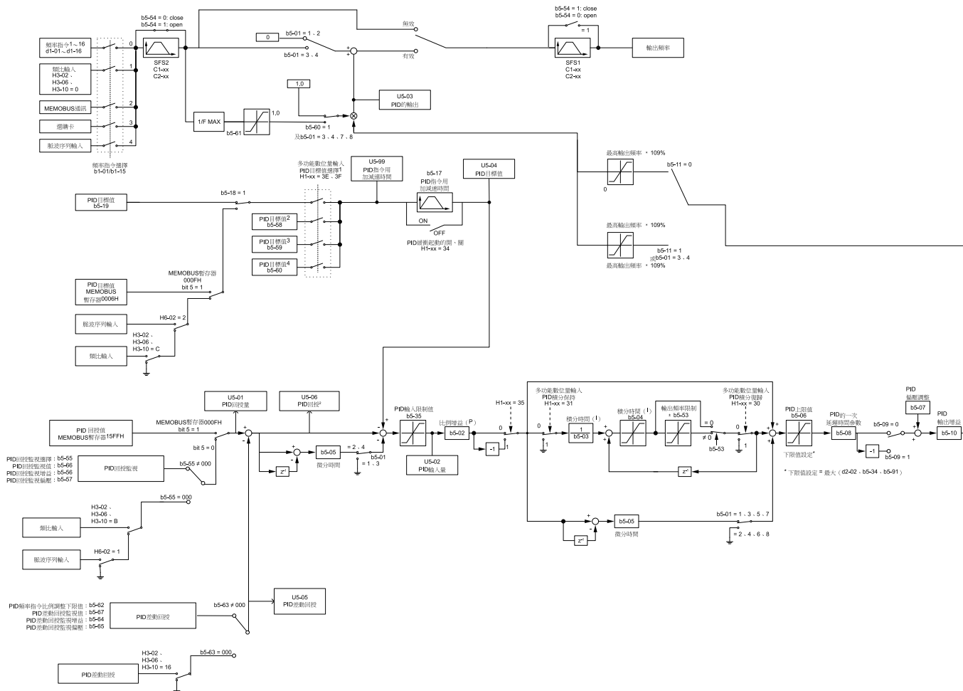
圖 11.35 PID控制區塊圖
