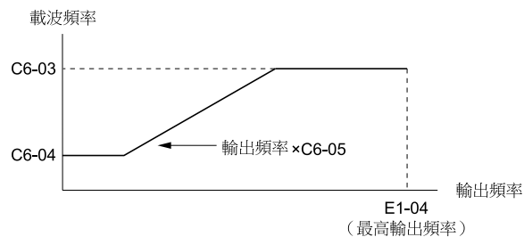
圖 11.55 與輸出頻率相應的載波頻率的變化
