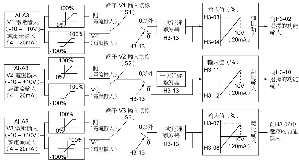
圖 11.71 類比輸入指令的單獨輸入區塊圖
