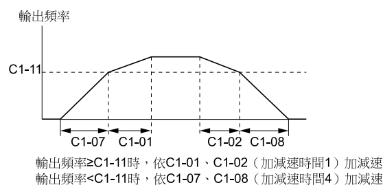
圖 11.45 加減速時間的切換頻率
