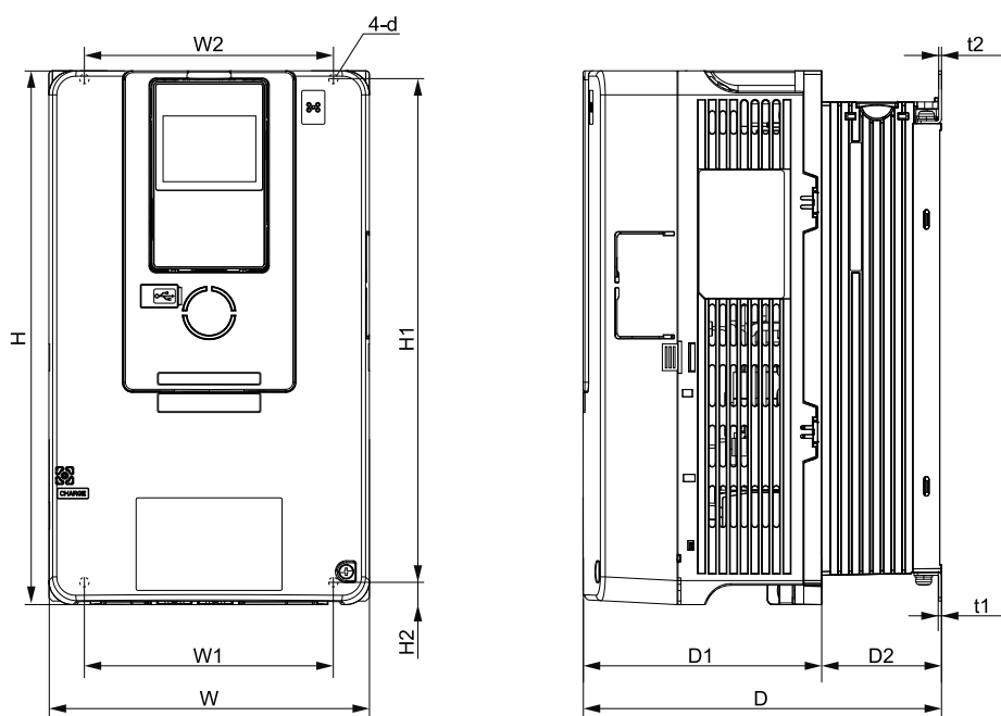
圖 9.2 外形圖2 (型號：2056、4031、4038)
