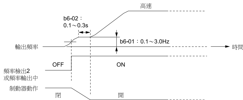
圖 11.6 起動時的DWELL功能
