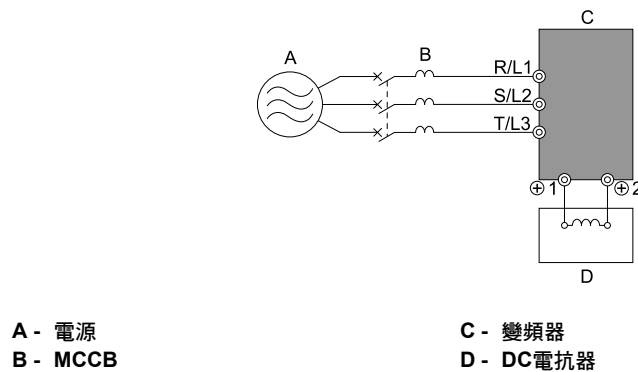
圖 2.67 DC電抗器的連接範例
