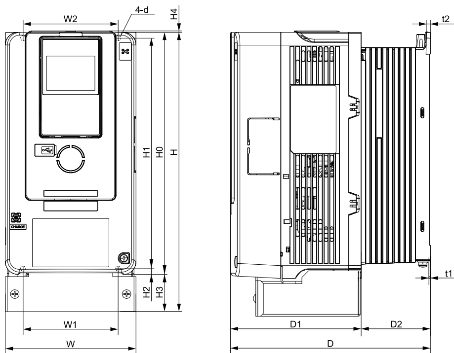
圖 9.3 外形圖1 (型號：2004~2042、4002~4023)
