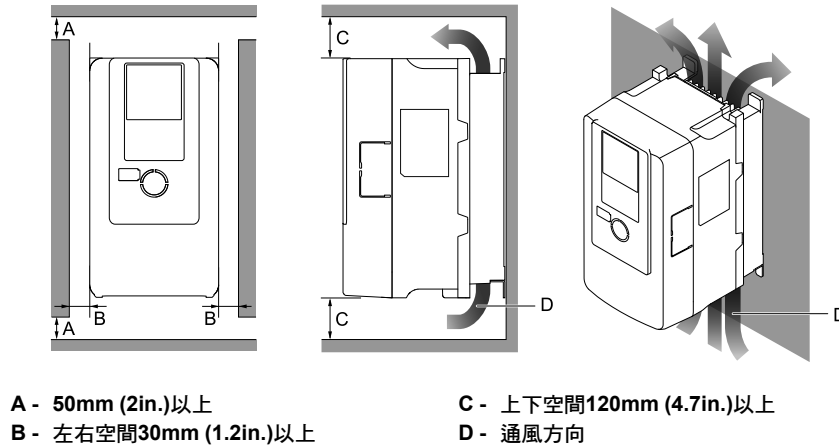
圖 2.2 變頻器的安裝空間 (單機)
