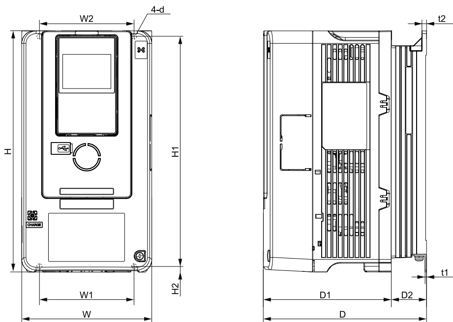
圖 9.1 外形圖1 (型號：2004~2042、4002~4023)
