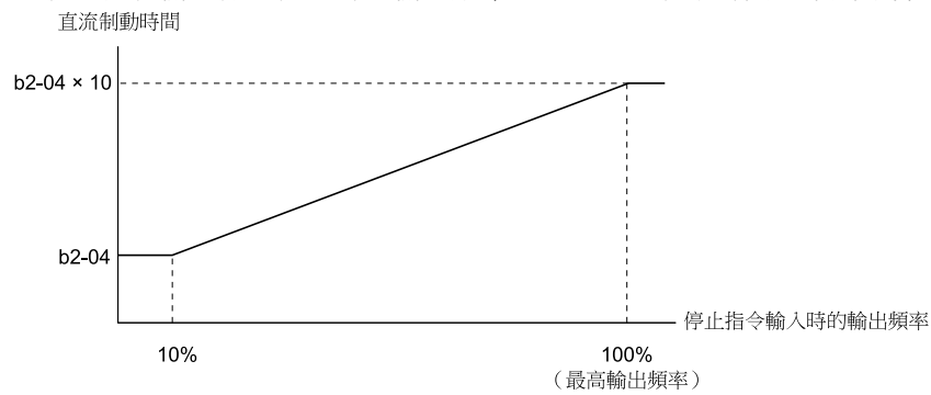
圖 11.14 全領域直流制動停止
