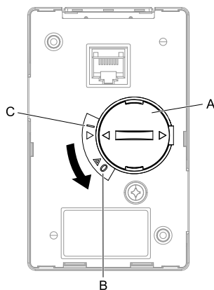
A - 電池蓋 B - 開啟 C - 關閉
