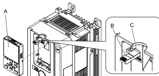
C - 插座
