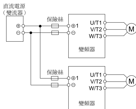
圖 4.3 直流電源輸入時的配線範例
