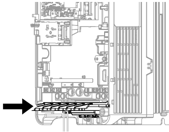
圖 7.26 安裝配線蓋
