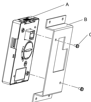
A - 操作器 B - 安裝配件A C - M3螺絲
