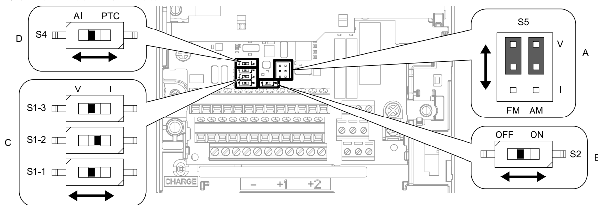
圖 2.52 開關排列
