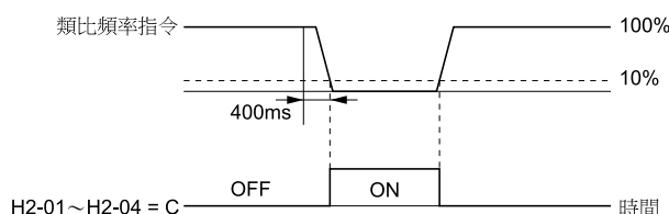
圖 11.133 頻率指令喪失的檢出
