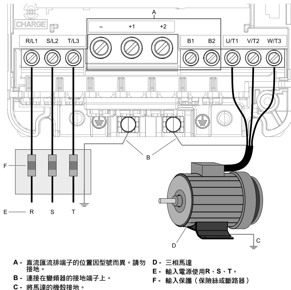
圖 2.29 將主迴路和馬達配線
