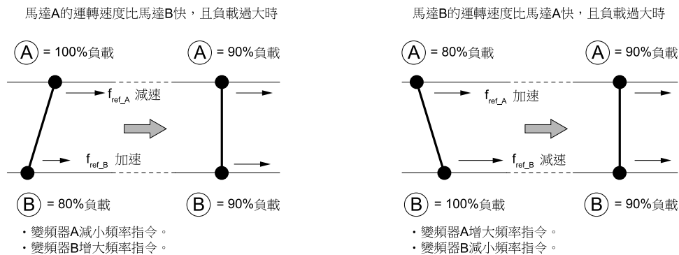
圖 11.41 DROOP控制（以起重機移動動作的俯視圖為例）
