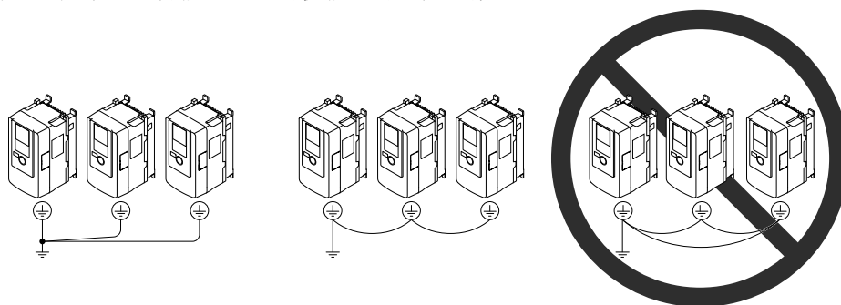
圖 2.32 多台變頻器的配線
