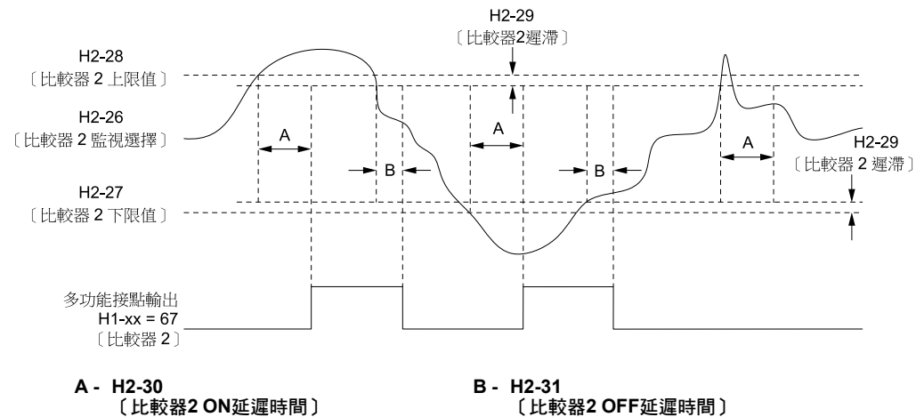
圖 11.98 比較器2輸出的時序圖
