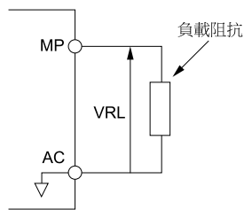
圖 11.113 作為共集極輸出使用時的迴路圖
