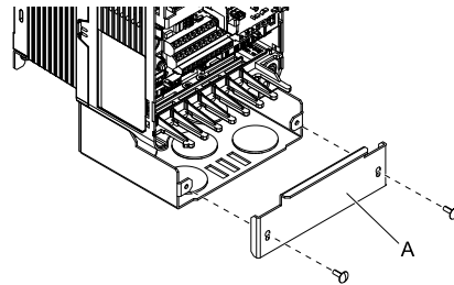
圖 2.26 安裝下部保護蓋2
